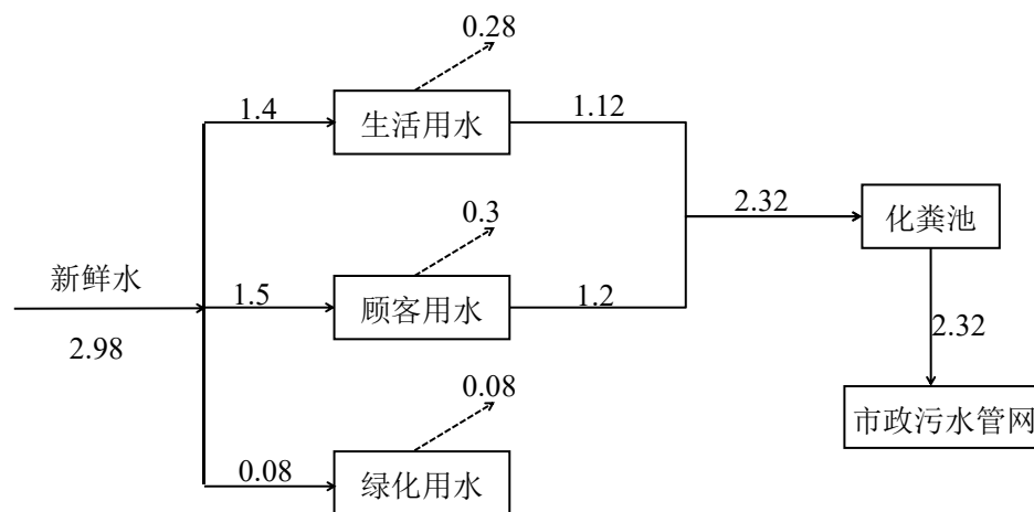
图 2-1 项目水平衡图 ( \text{m}^3/\text{d} )
