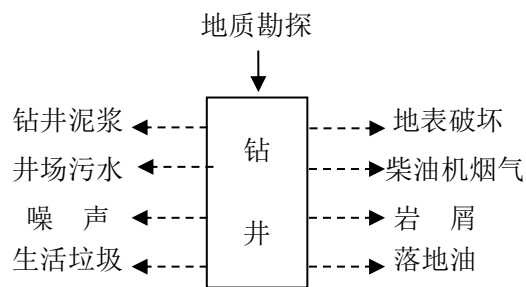
图 4-2 钻探井工艺流程及产污节点图
